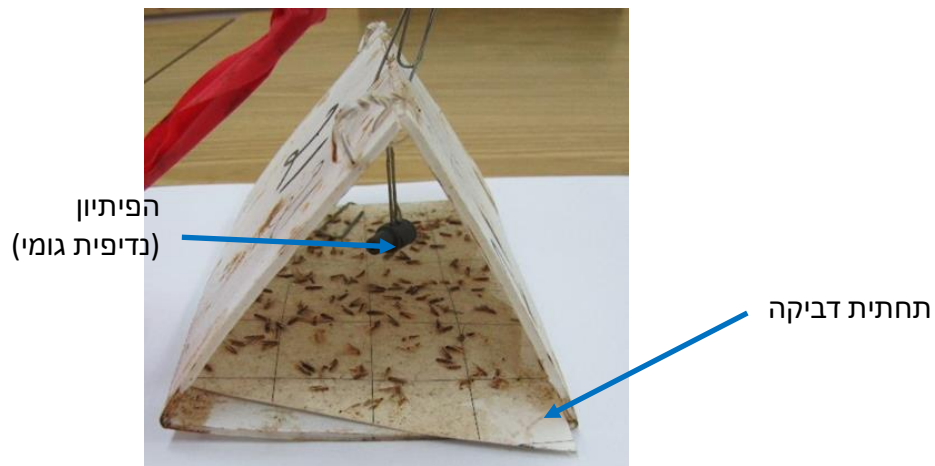
מלכודת דלתא מסוג "ג'קסון"
